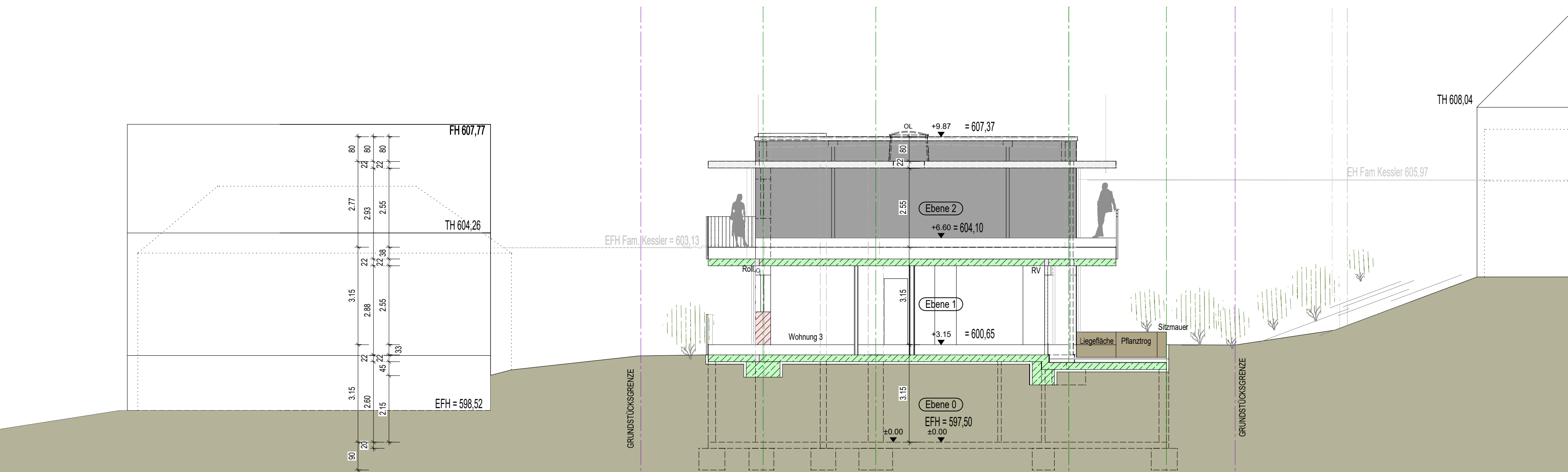
Schnittansicht 4
