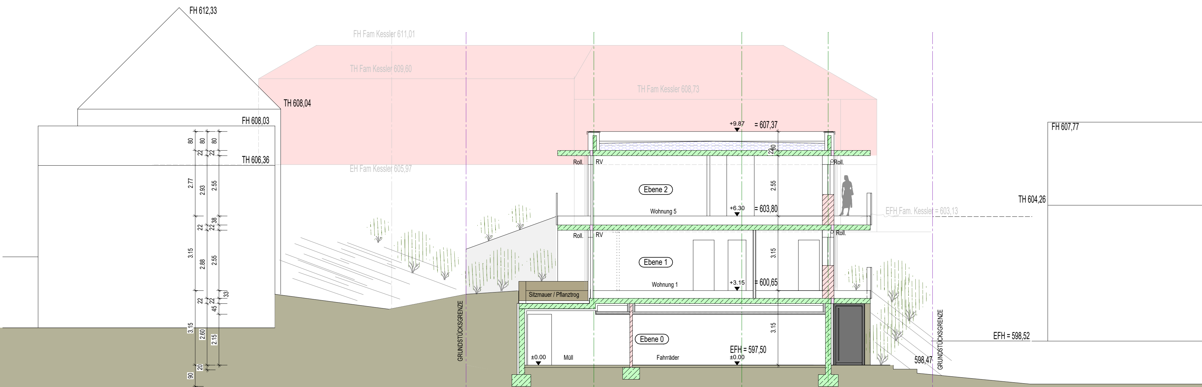
Schnitt 2
